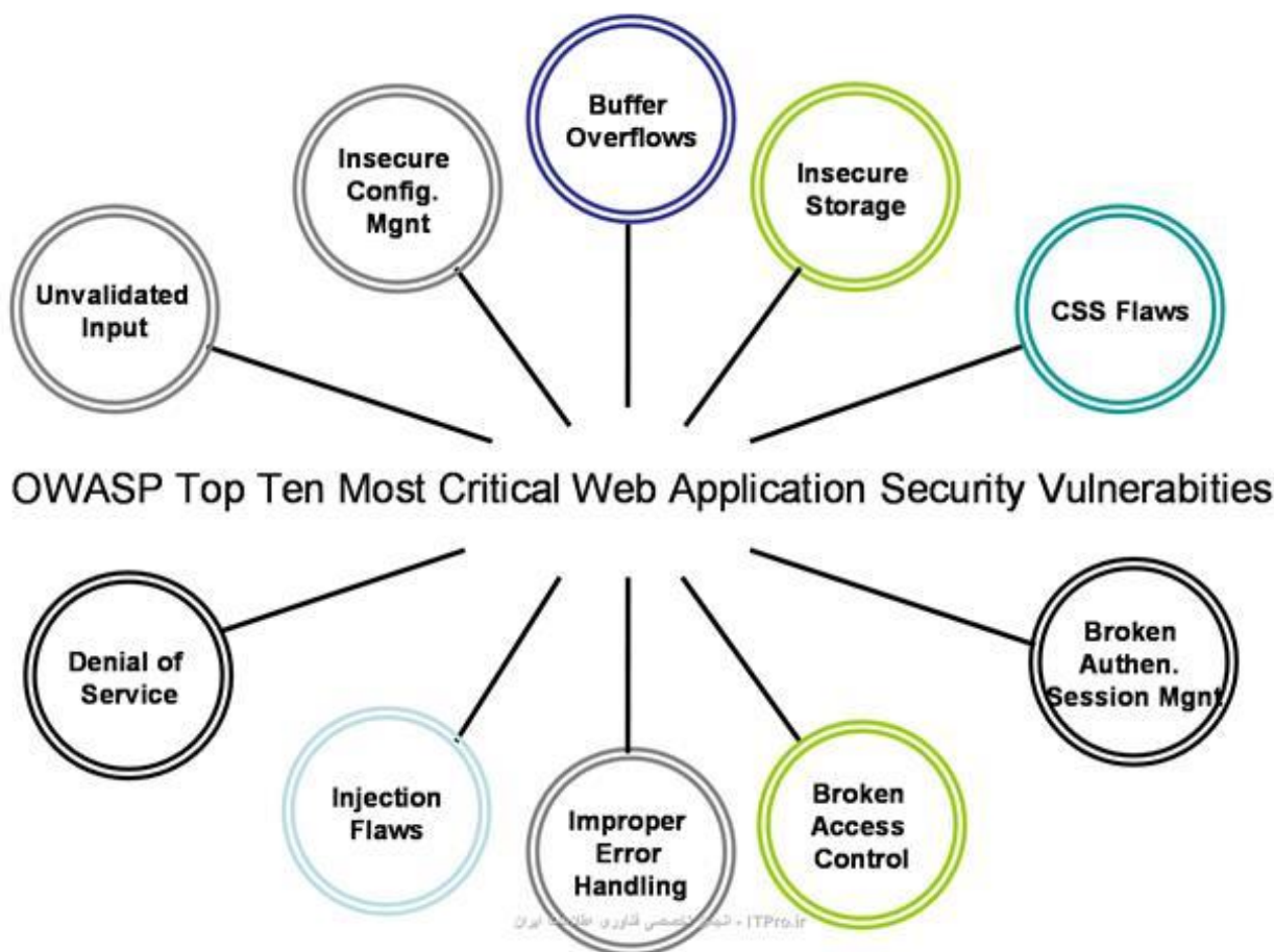
شکل ۴- پروژه OWASP
