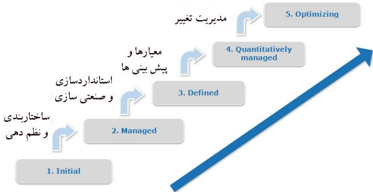
شکل ۴- سطوح CMMI
